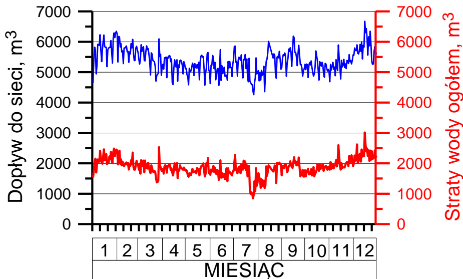
Rysunek 1 – Wykres ilości wody wtłoczonej i traconej w całym systemie wodociągowym, w 2020 r.
