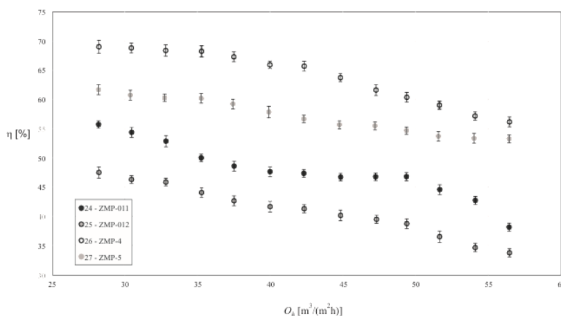
Rysunek 1. Stopień separacji cząstek stałych lekkich w wodzie w zależności od obciążenia hydraulicznego dla zmodyfikowanych osadników wirowych z przegrodą wzdłużną.
