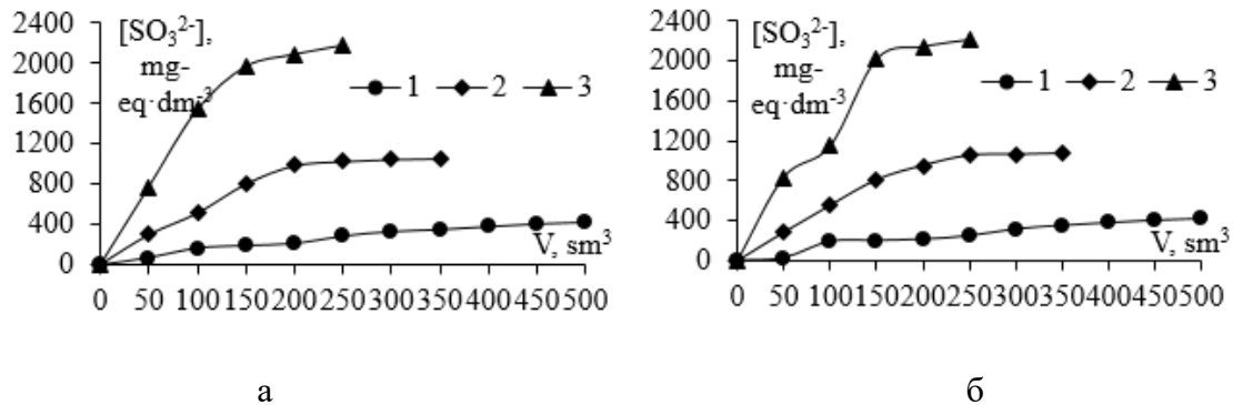
Рисунок 1 – Залежність концентрації сульфитів (1; 2; 3) від пропущеного об’єму розчину метабисульфиту натрію концентрацією, %: 2 (1); 5 (2); 10 (3), через аніоніт АВ-17-8 в СГ-формі (а) та основній формі (б) ( V_i=20 \text{ см}^3 ) (ПОДС 1 =3515 мг-екв·дм -3 ; ПОДС 2 =4167 мг-екв·дм -3 ; ПОДС 3 =5870 мг-екв·дм -3 )
