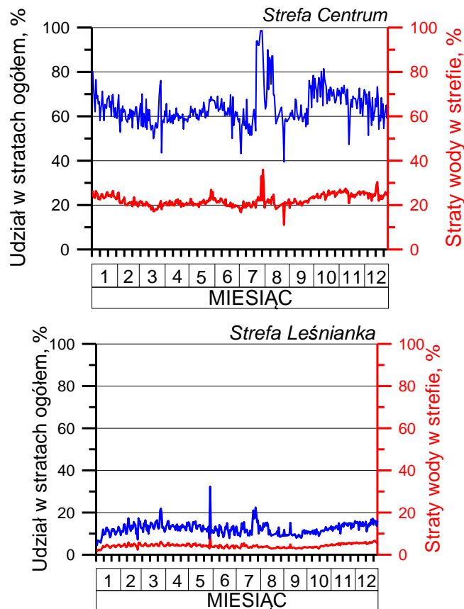
Rysunek 2 – Wykres dobowych strat wody w dwóch strefach o największych udziałach strat całego systemu w 2020 r. Dolna linia (czerwona) straty wody w strefie, linia górna (niebieska) udział wody traconej w strefie w stosunku do strat wody w całym systemie
