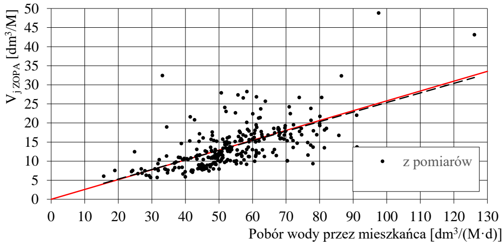
Rysunek 3 – Obliczona pojemność jednostkowa ZOPA w zależności od jednostkowego poboru ciepłej wody we wszystkich budynkach dla wszystkich dni pomiarowych
