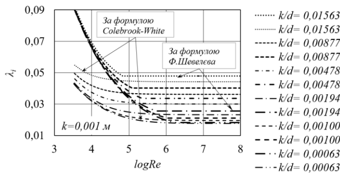
Рисунок 1 – Закономірності зміни параметра \lambda_i , обчисленого за методиками Ф.Шевелєва і Colebrook-White в залежності від параметра Re для різних значень відносної шорсткості внутрішньої поверхні труб k/d
